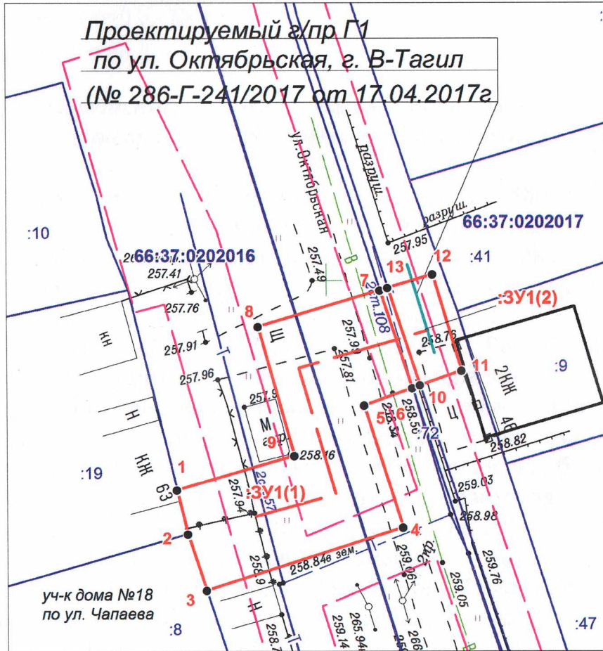
Масштаб 1:500
