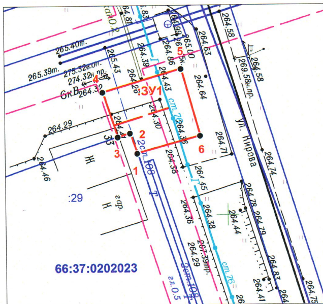
Масштаб 1:500
